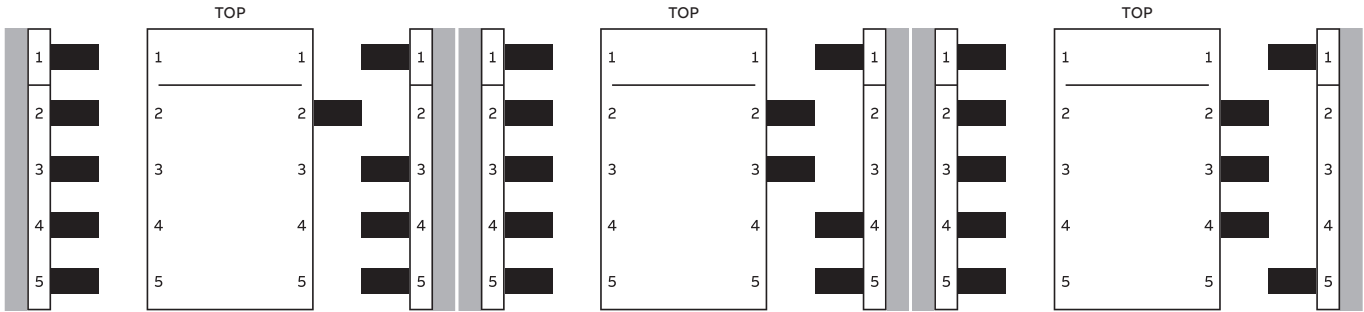
ANSI BR 800, E 85 kA SQ
