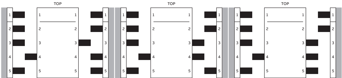
ANSI BR 800, S 65 kA
