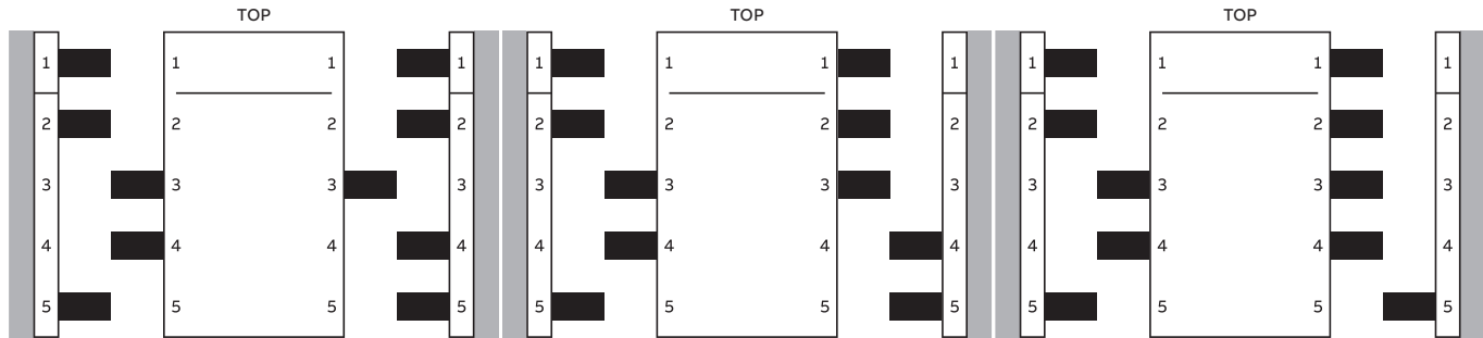
ANSI SW 800, M 65 kA
