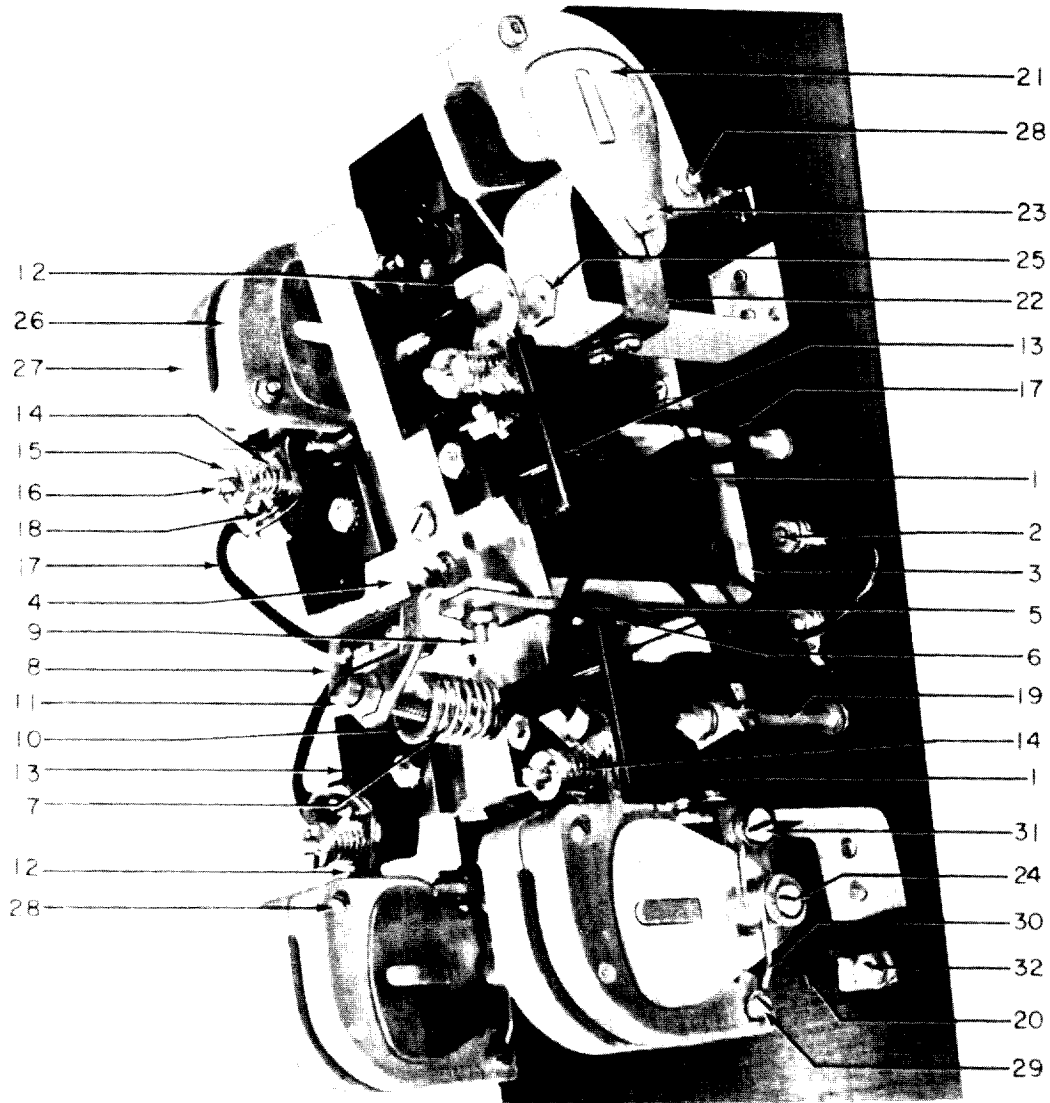
IC2800-A122-A contactor
